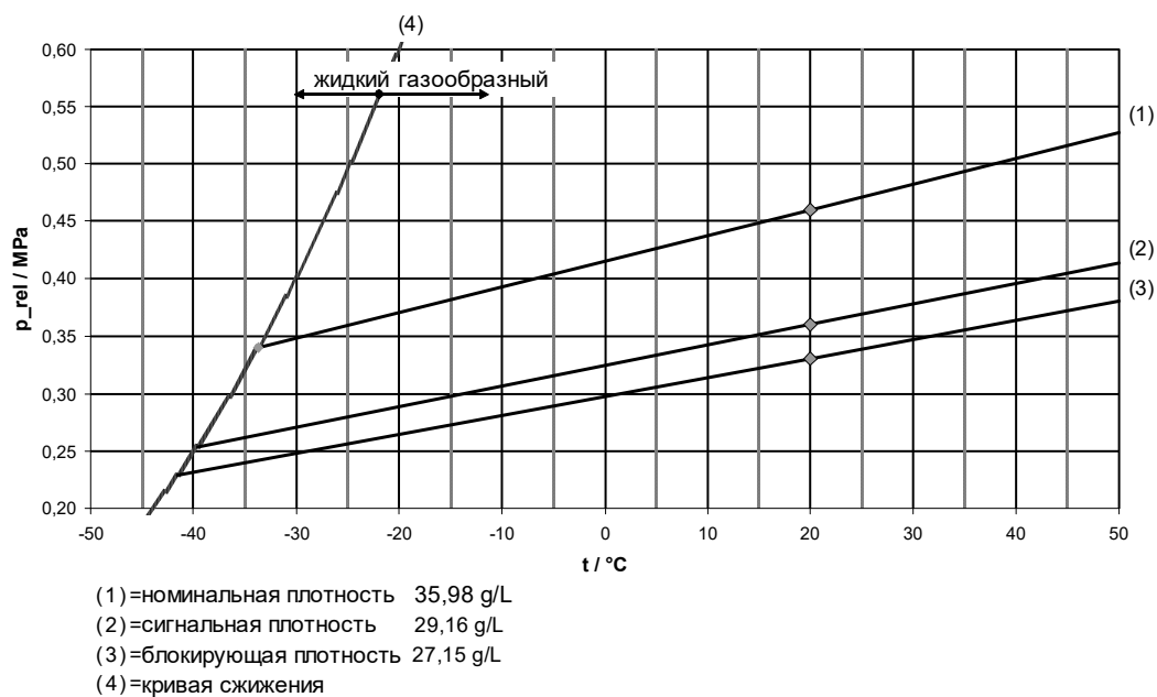
Кривая давления элегаза -40°C (ND=0,46 МПа [p e ] / UW1=0,36 МПа [p e ] / UW2=0,33 МПа [p e ])
